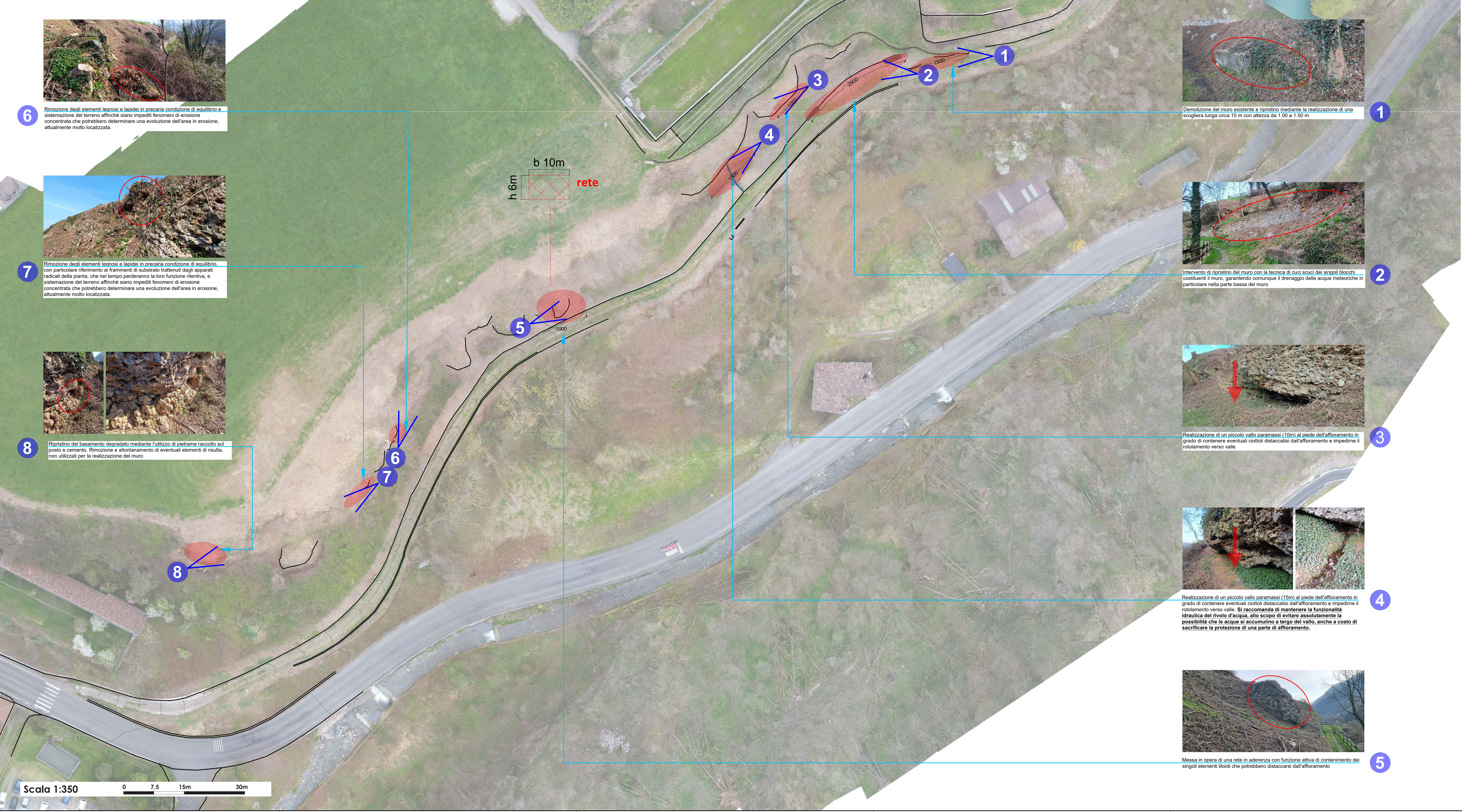
Tav. Inquadramento interventi per la messa in sicurezza di via Carducci
