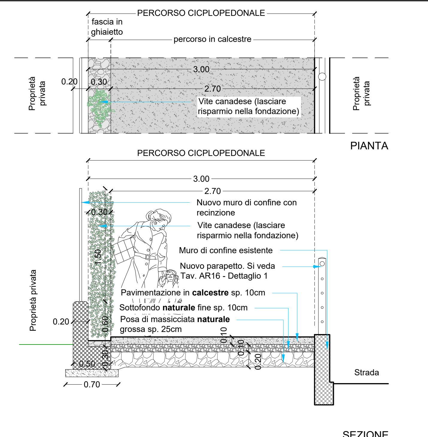
PIANTA E SEZIONE B Scala 1:30
