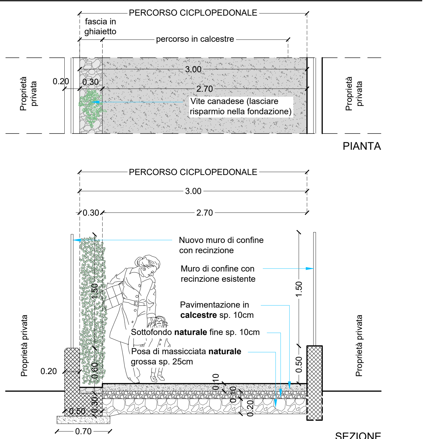
PIANTA E SEZIONE C Scala 1:30
