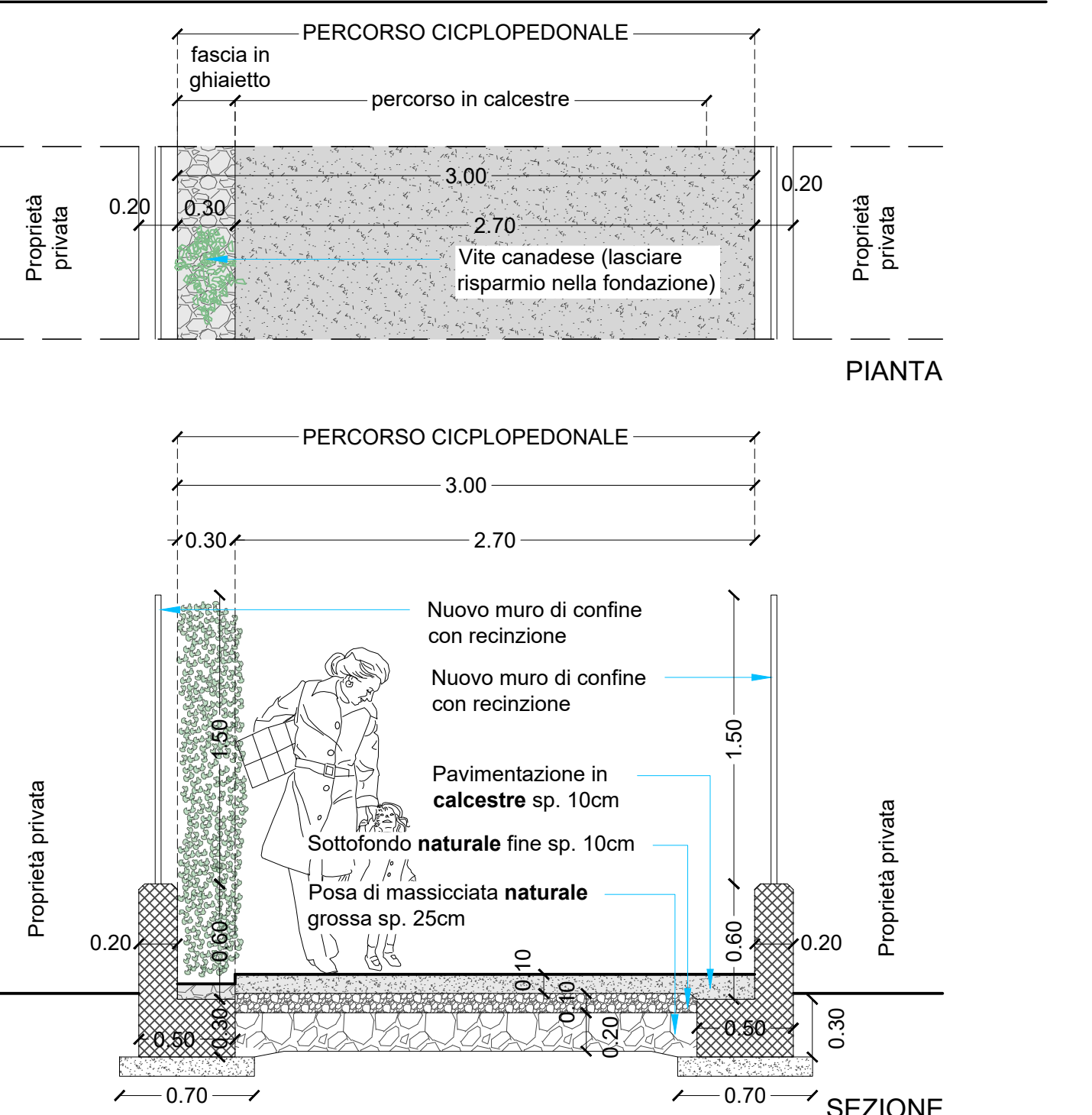
PIANTA E SEZIONE D Scala 1:30
