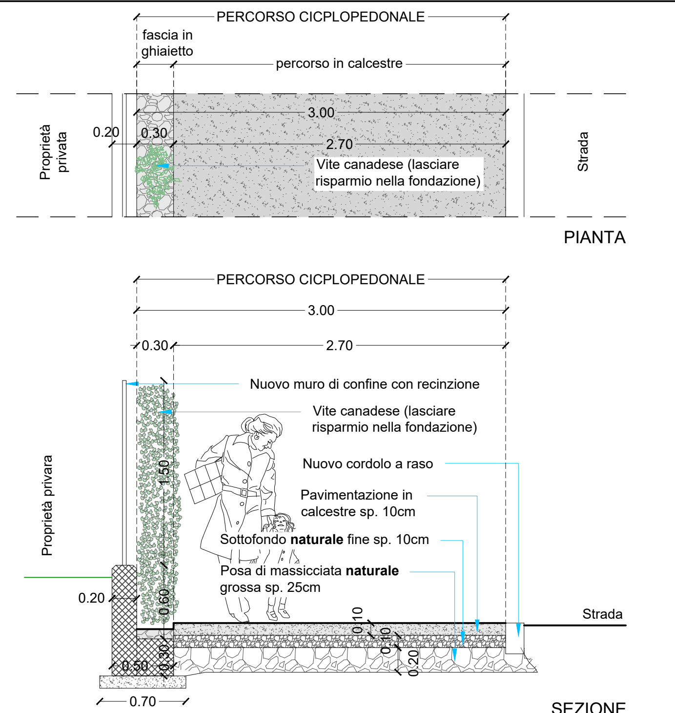
PIANTA E SEZIONE A Scala 1:30
